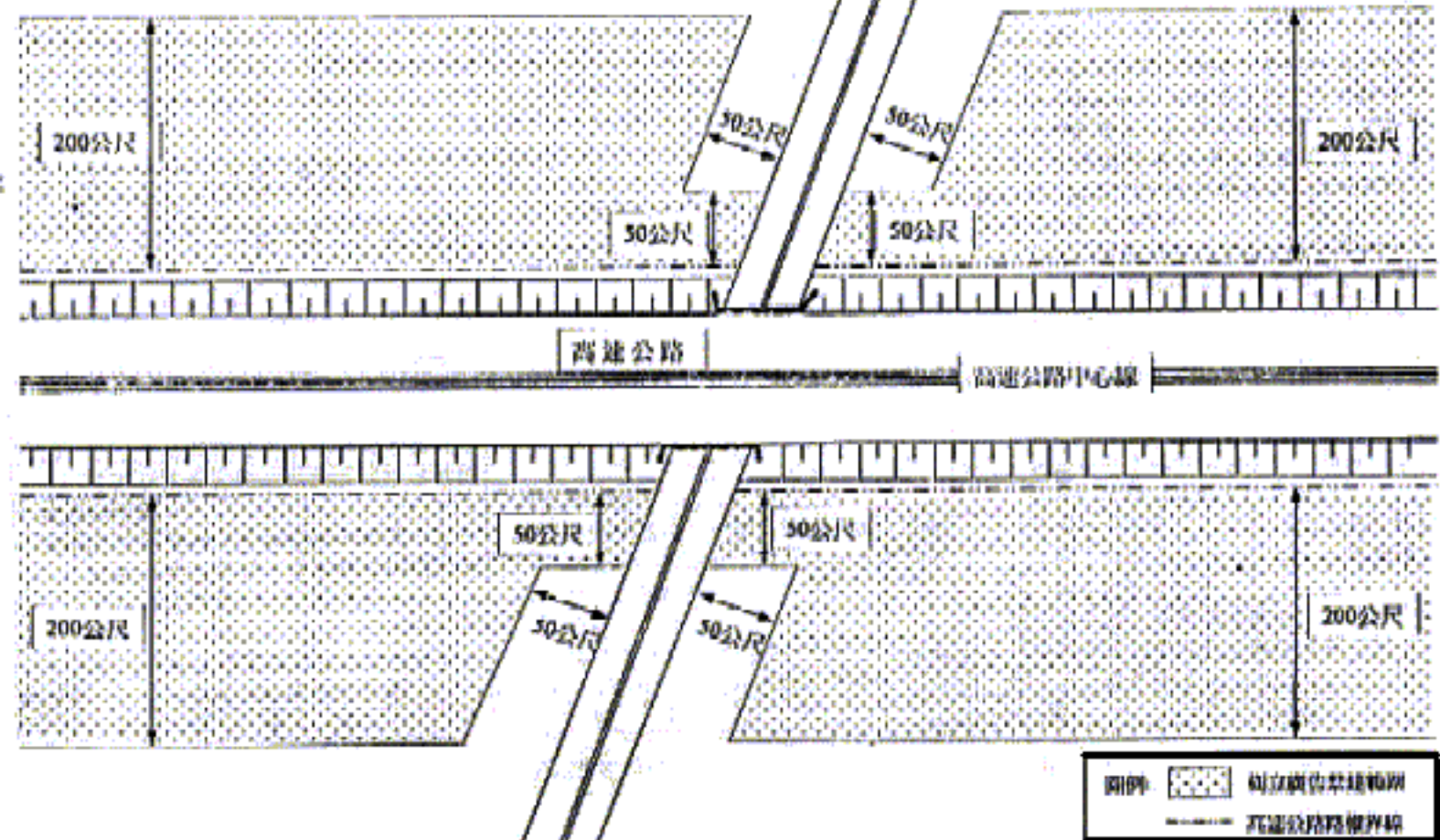
圖二 高速公路與省道或市道、縣道立體交會路段樹立廣告禁建範圍示意圖
