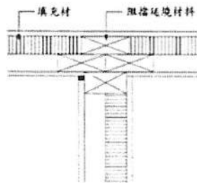
圖9.3-5 防火被覆用板材接縫部分與阻擋延燒材料示意圖範例（一）
