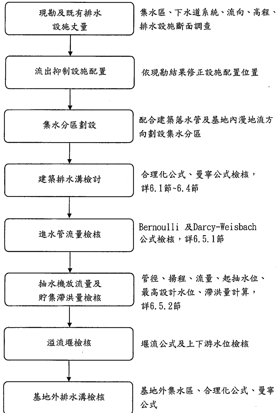
圖 6.1 設計流程圖
