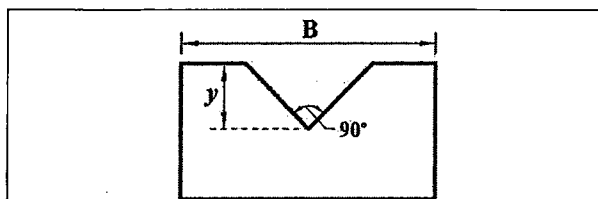
直角三角堰
