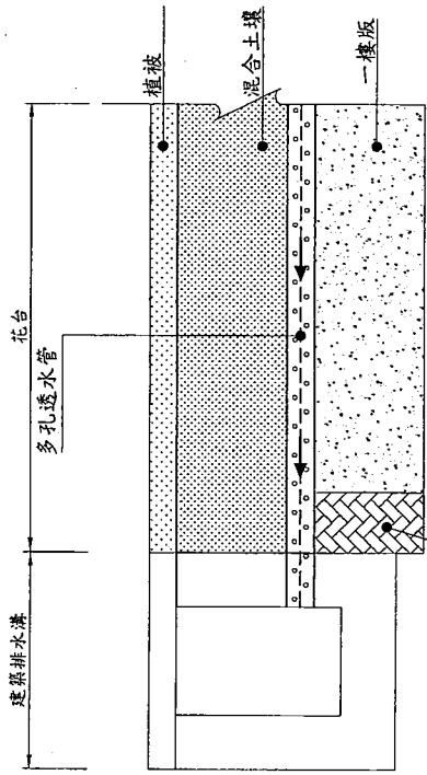
花台透水管配置示意圖 (B-B) 1/10 unit:cm
