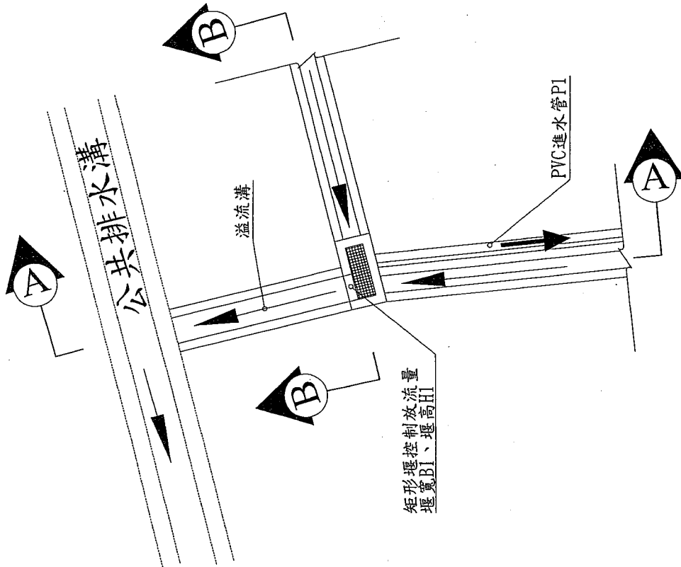
矩形堰B1及溢流溝平面圖(一) 1:40 unit:cm
