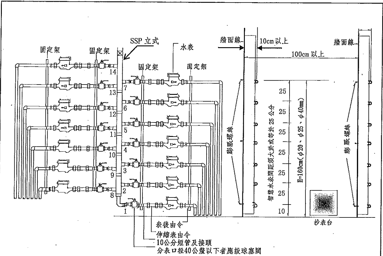
水表固定架側視圖
