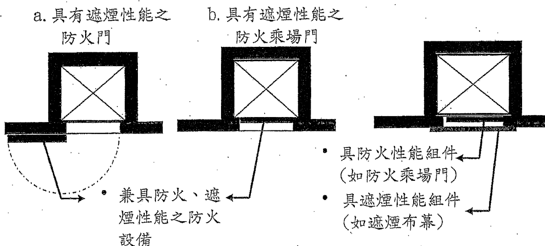
圖一、單一型防火設備
